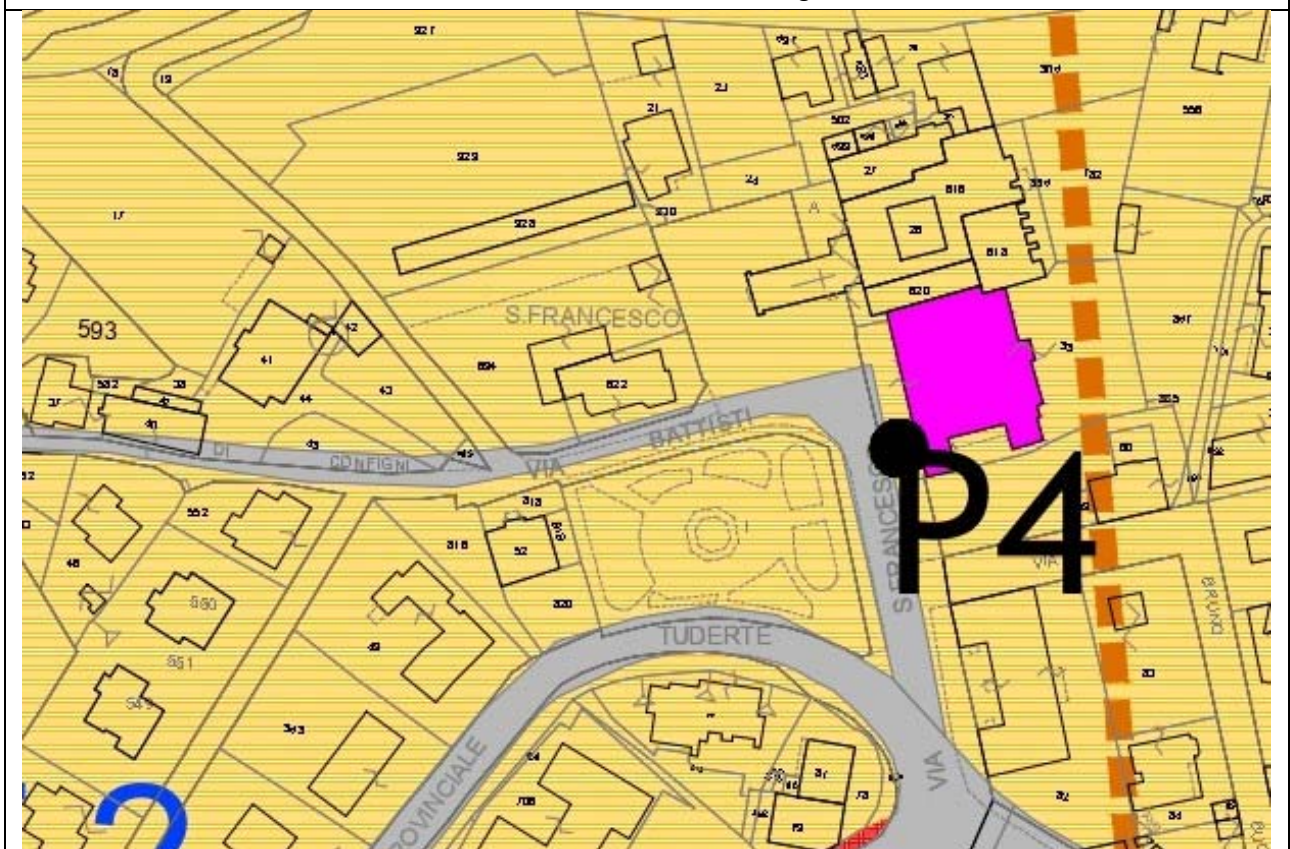
Punto di misura P4: individuazione su PCCA
