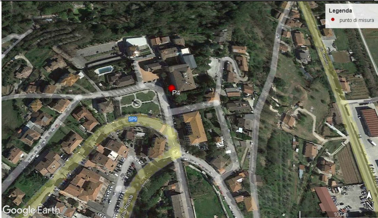
Punto di misura P4: individuazione su foto aerea
